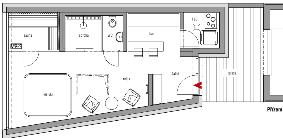
Objekt relaxu v návaznosti na bazénu a stávající rodinný dům
